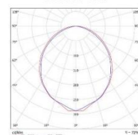
Curva Polar
